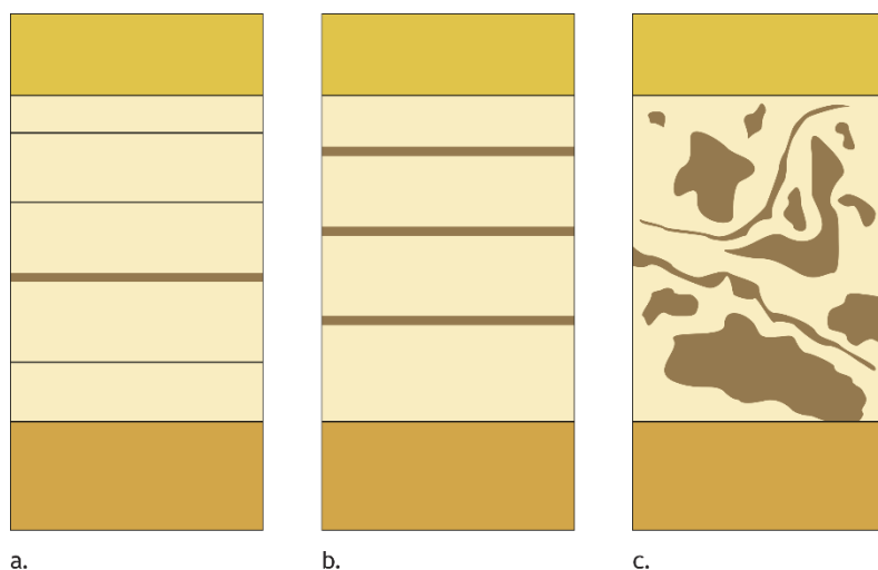
Figuur 5: De lichtgekleurde laag stelt een eenheid voor die uit een andere grondsoort bestaat dan de aangrenzende lagen. In het eerste geval (a) wordt de laag als een homogeen geheel beschreven met daarin een afwijkend laagje. In het tweede geval (b) wordt de laag beschreven als opgebouwd uit laagjes die in grondsoort verschillen. In het derde geval (c) wordt de laag beschreven als opgebouwd uit laagdelen die in grondsoort verschillen.
