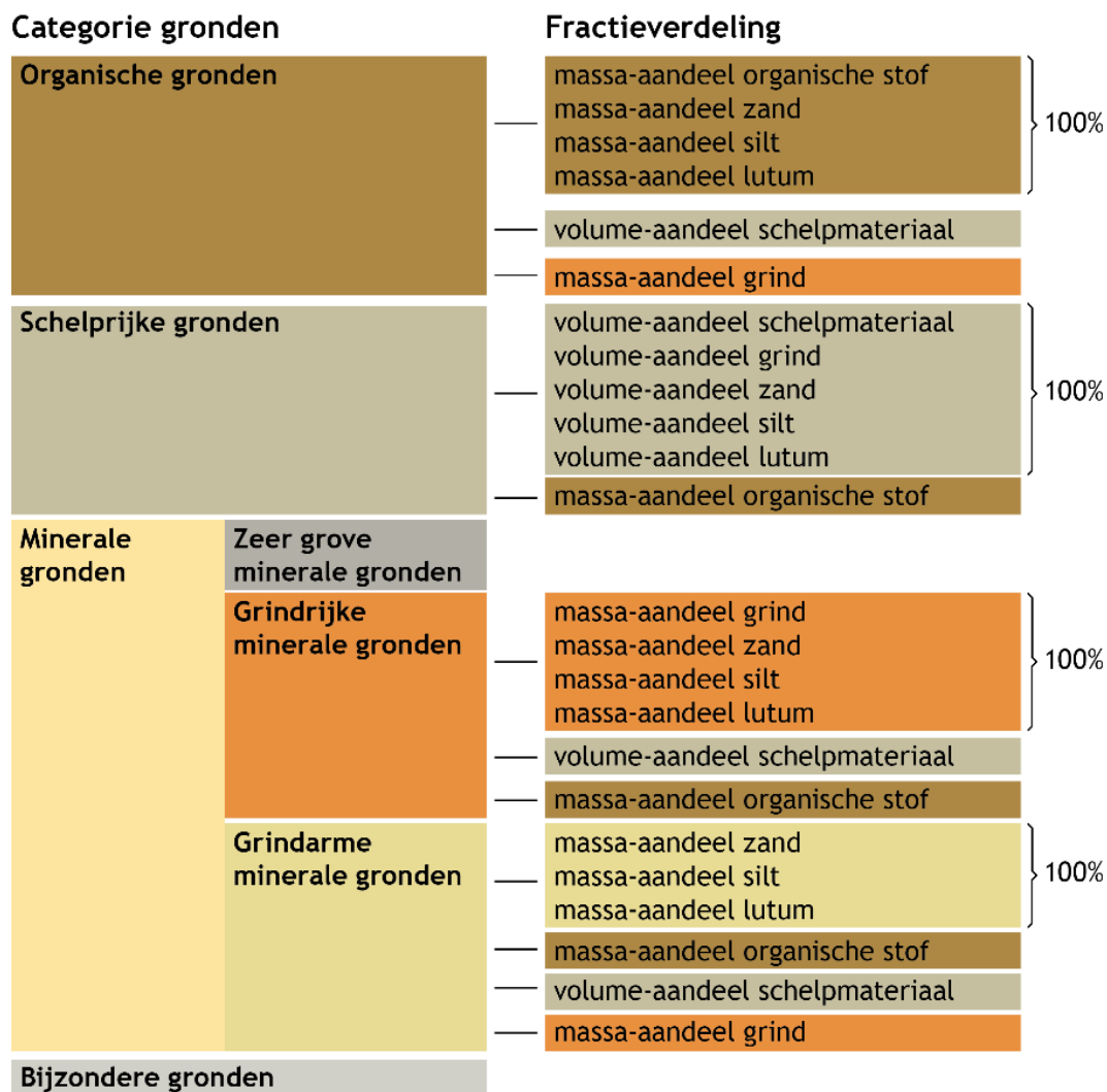
Figuur 6: Er worden zes categorieën grond onderscheiden. Van zeer grove minerale gronden en bijzondere gronden wordt geen fractieverdeling bepaald, van de andere wel. Per categorie grond is in kleur aangegeven welke fracties tot 100 procent optellen. Voor verdere toelichting zie de tekst.
