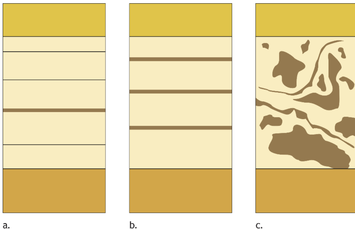
Figuur 5 De lichtgekleurde laag stelt een eenheid voor die uit een andere grondsoort bestaat dan de aangrenzende lagen. In het eerste geval (a) wordt de laag als een homogeen geheel beschreven met daarin een afwijkend laagje. In het tweede geval (b) wordt de laag beschreven als opgebouwd uit laagjes die in grondsoort verschillen. In het derde geval (c) wordt de laag beschreven als opgebouwd uit laagdelen die in grondsoort verschillen.
